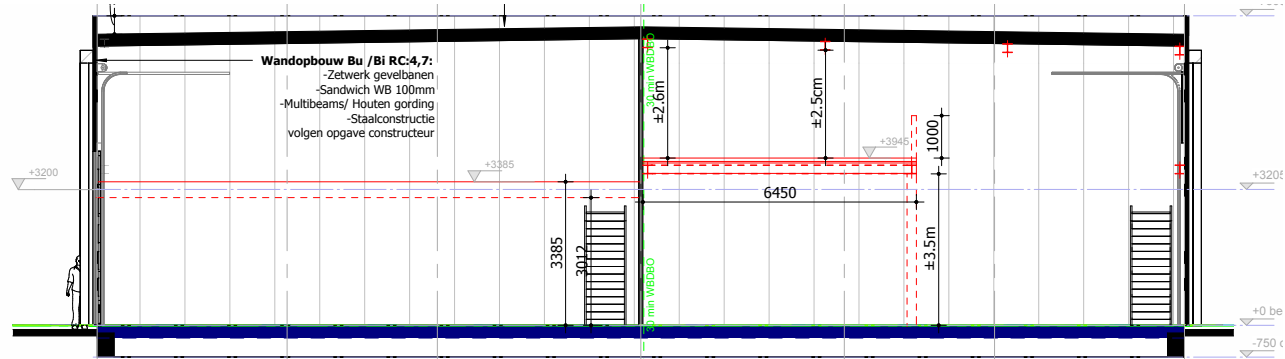
DOORSNEDE A
