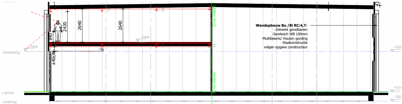
DOORSNEDE B
